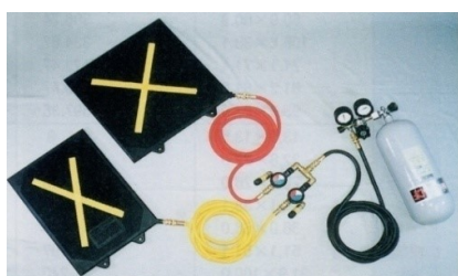
マット型空気ジャッキ
