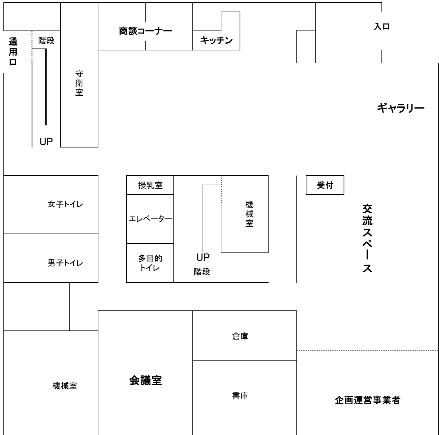
3階
