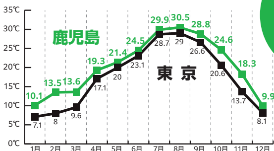
年間平均気温比較(令和6年) ※資料 気象庁
