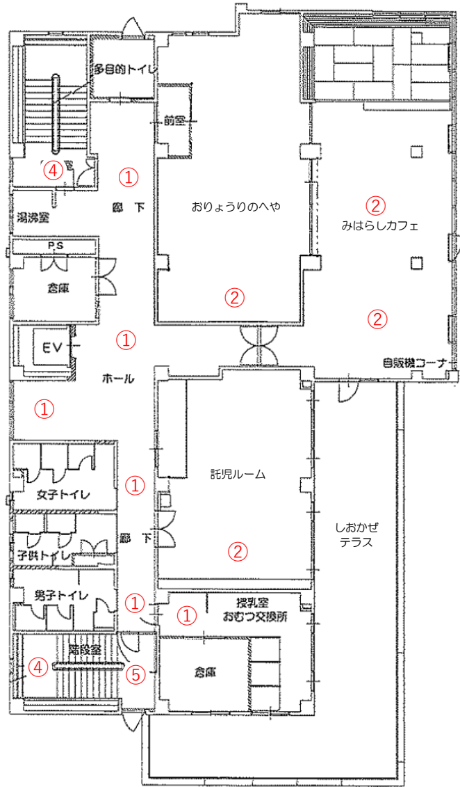
2階平面図
