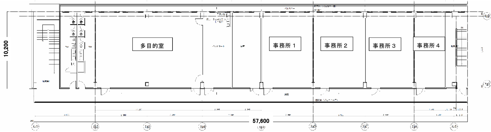
2階平面図
