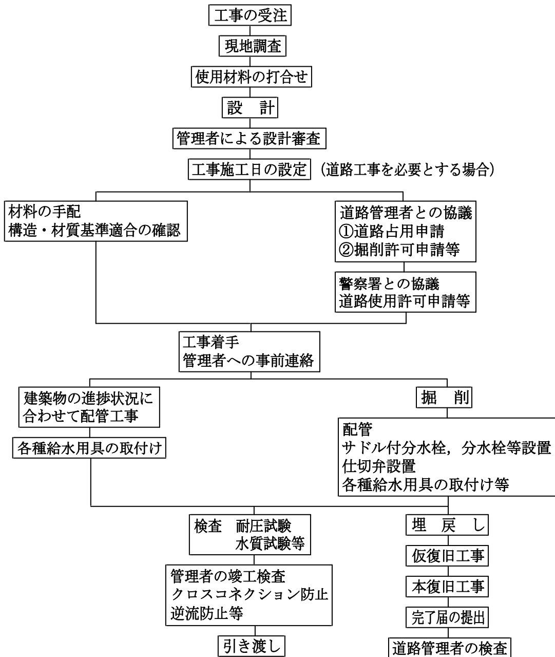
図1-1 給水装置工事の工程の例
