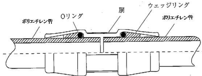
図 3 - 59 ワンタッチ式継手
