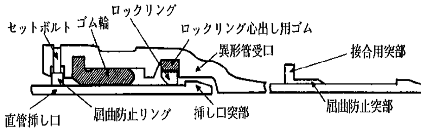
図 3 - 69 - 2 NS形異形管の継手接合
