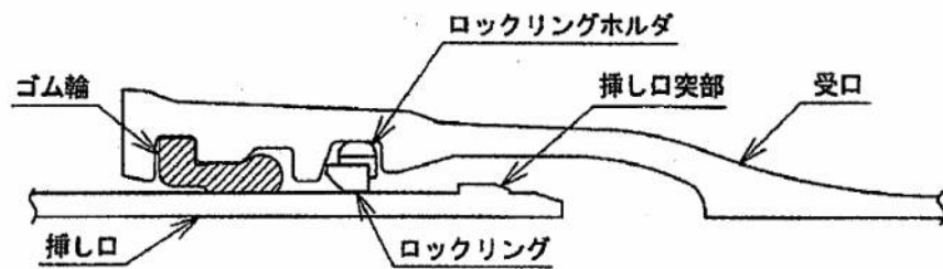
図 3 - 69 - 3 GX形直管の継手接合
