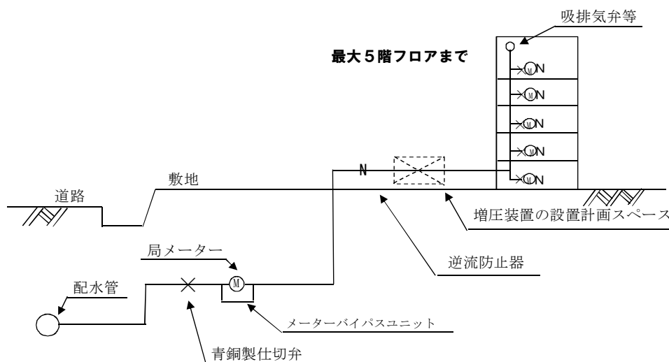
図3-3-2 特例直結直圧式
