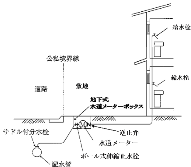
図 3 - 1 直結直圧式の一般図
