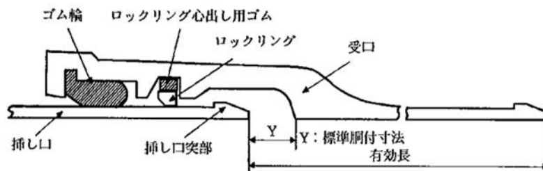
図 3 - 69 - 1 NS 形直管の継手接合
